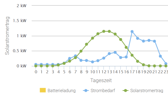
Abbildung: Solarstromertrag und -bedarf im Tagesverlauf (Quelle: Solardachkataster RVR)
